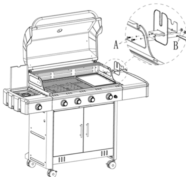
۲- سرهم‌بندی نگه‌دارنده
