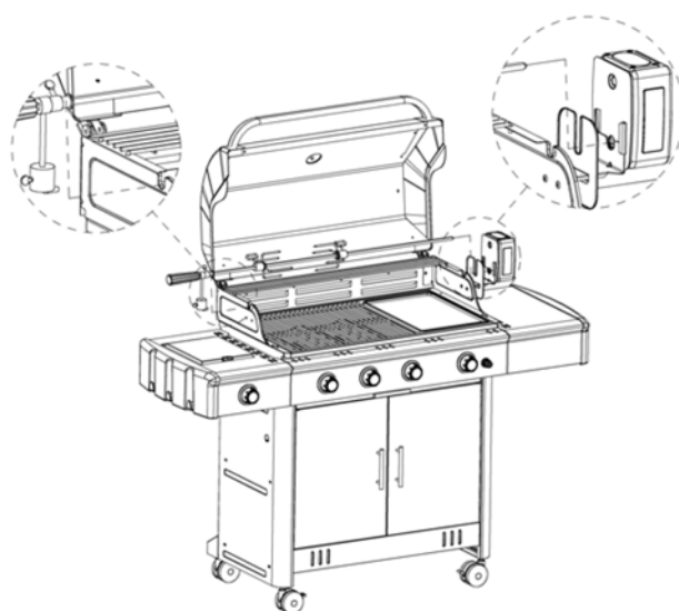
۴- سرهم‌بندی جوجه‌گردان
